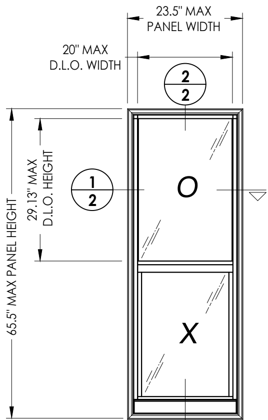
DLP LITE FRAME WINDSERT™
