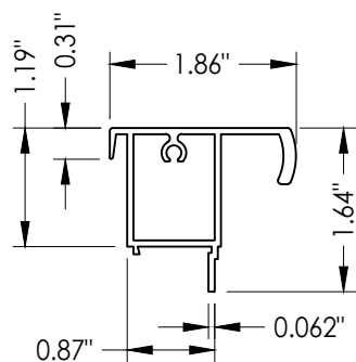
2E VENT TOP RAIL ALUM (6063-T6)
