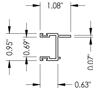
2J VENT JAMB ALUM (6063-T6)
