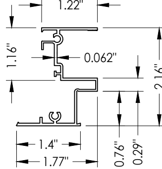
2H FRAME JAMB ALUM (6063-T6)
